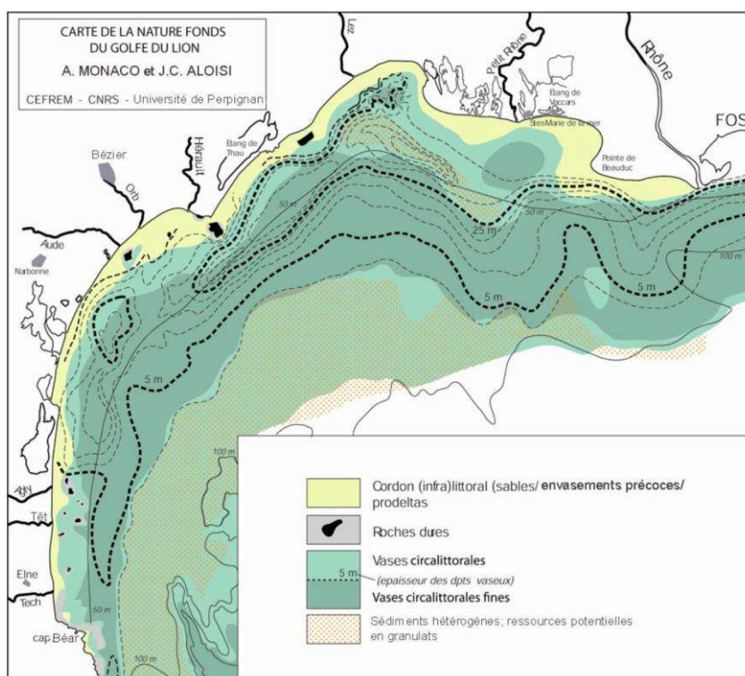
Figure 22 : Carte sédimentologique du golfe du Lion (Aloisi, 1973 in Labruno, 2006)
