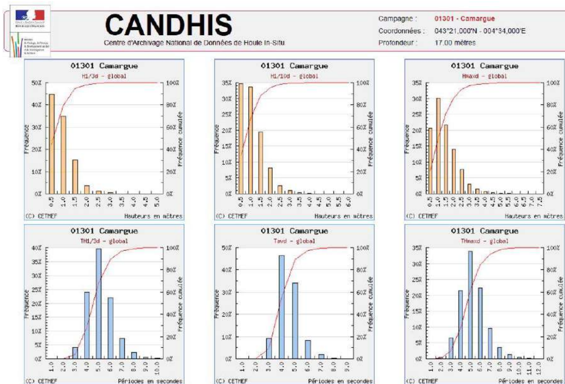
Figure 16 : Données de houle de la bouée Camargue de 1999 à 2004 (source CANDHIS).
