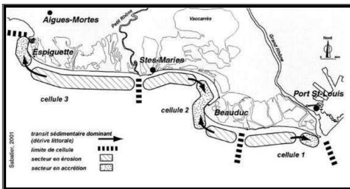
Figure 21 : Transport et cellules sédimentaires en Camargue (Sabatier, 2001)
