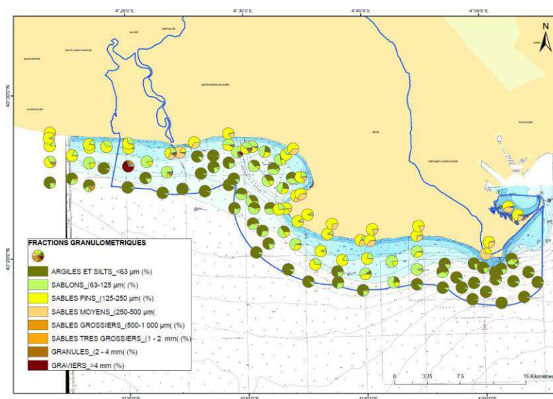
Figure 24 : Fractions granulométriques des 83 stations prospectées dans le cadre de l'étude CARTHAM (source : In Vivo, 2012)
